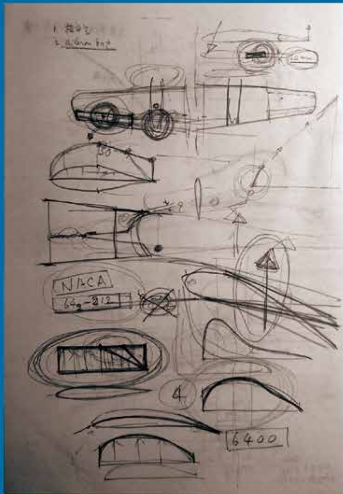
国産旅客機YS-11の基礎設計で構造を担当した堀越二郎の主翼検討スケッチ（本資料の実物展示はありません）
